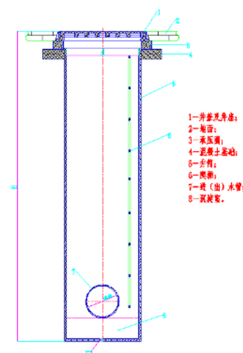
图1.直壁井示意图（ \Phi \leq 800 ）
