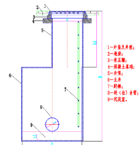
图2.收口井示意图（ \Phi > 800 ）
